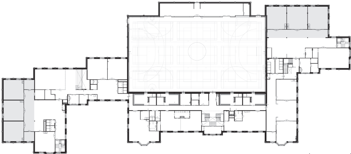
begane grond
