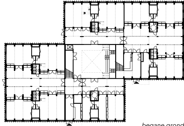
begane grond
