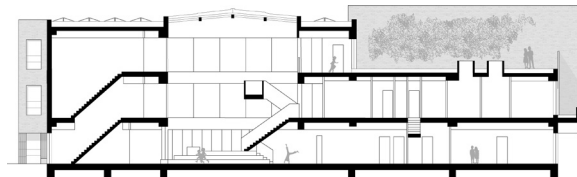
doorsnede
