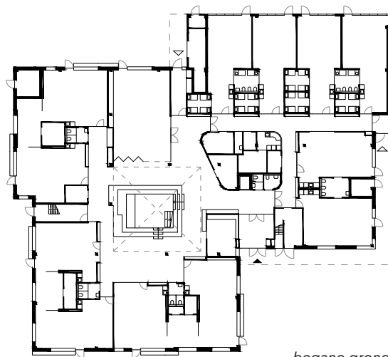
begane grond
