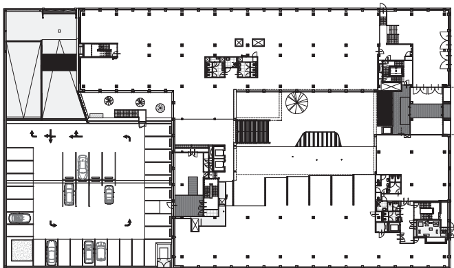
begane grond
