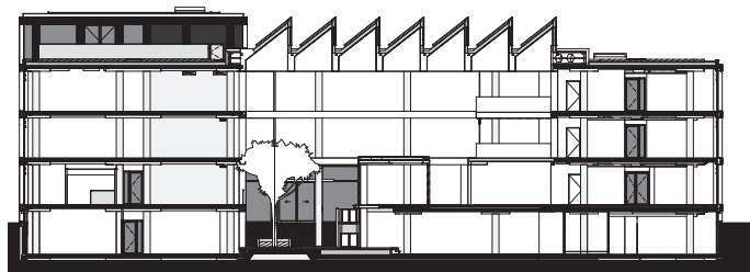
doorsnede
