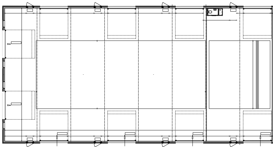
plattegrond
