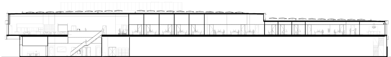
doorsnede
