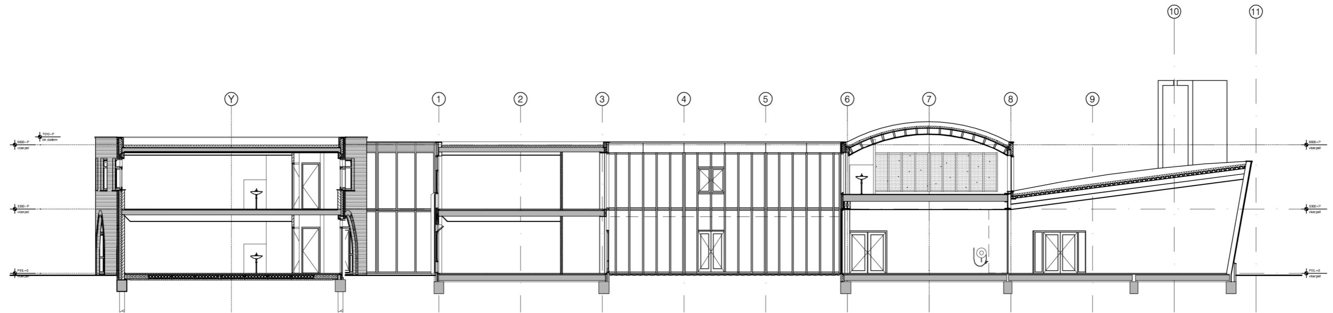
DOORSNEDE A-A
