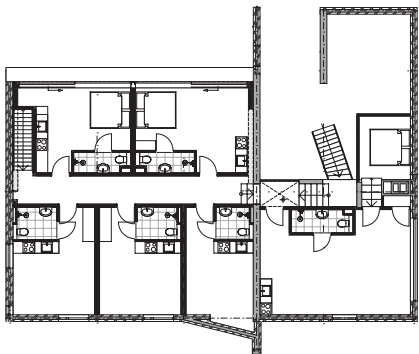
eerste verdieping
