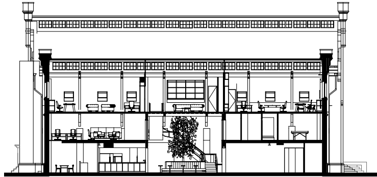
doorsnede
