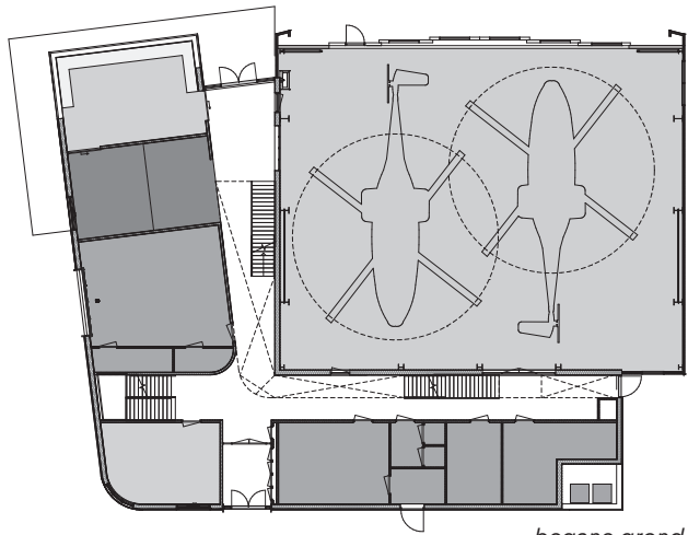
begane grond
