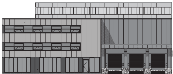
voorgevel
