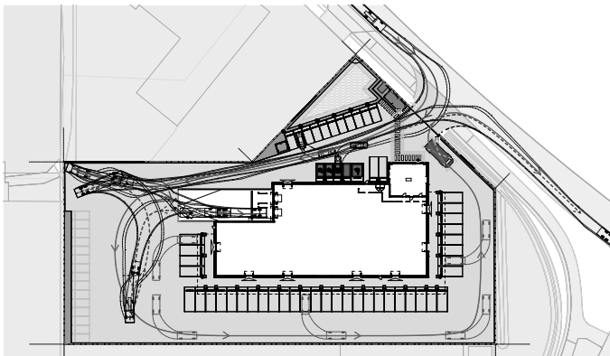
situatie met begane grond
