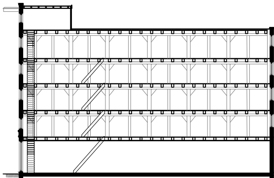
doorsnede
