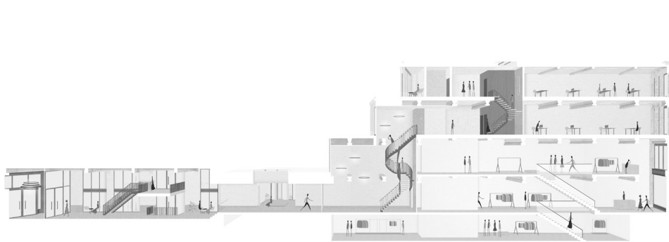
doorsnede
