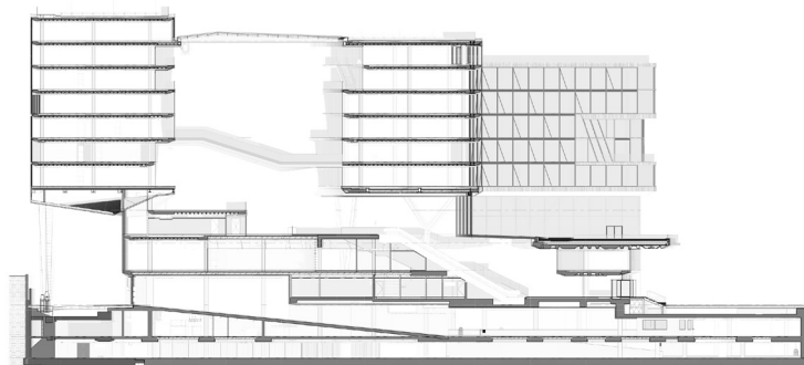
zijgevel
