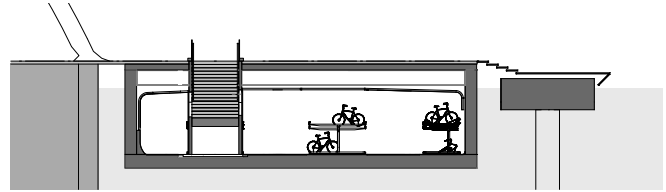
doorsnede
