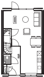
begane grond
