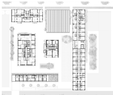
situatie met begane grond
