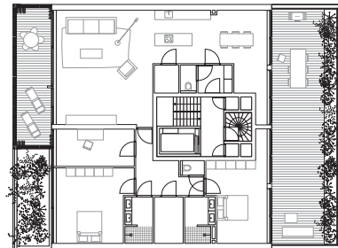
vijfde verdieping
