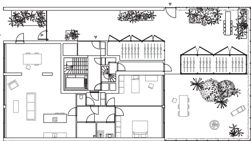
begane grond
