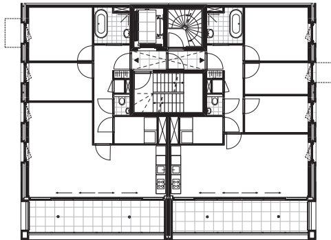
eerste t/m vierde verdieping
