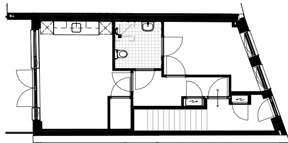
woningplattegrond Derde Oosterparkstraat 242H
