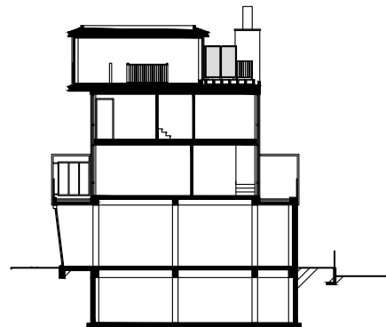
doorsnede
