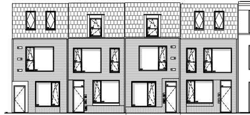
voorgevel
