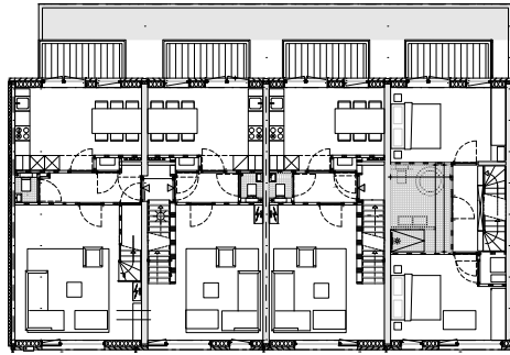
eerste verdieping
