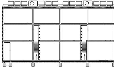
doorsnede
