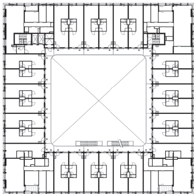
derde verdieping
