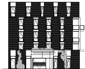
zuidoostgevel
