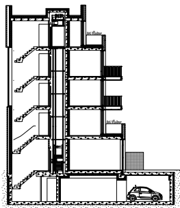
doorsnede
