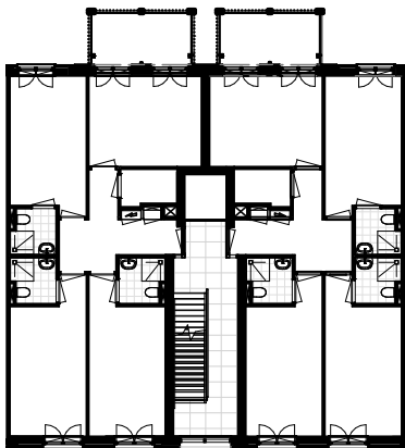
woningplattegronden eerste verdieping
