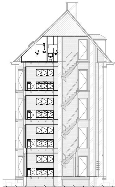
doorsnede
