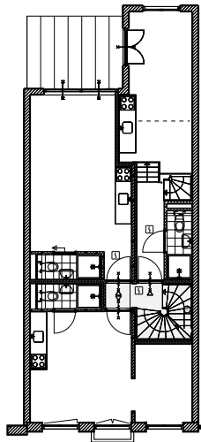
eerste verdieping
