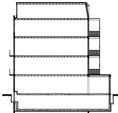
doorsnede
