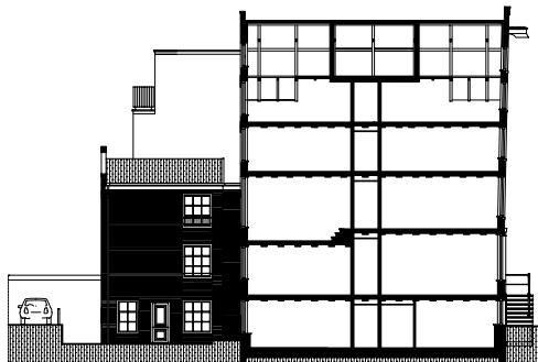
doorsnede
