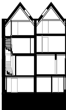
doorsnede
