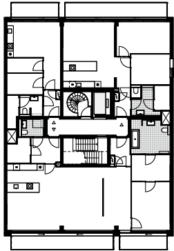
vijfde verdieping
