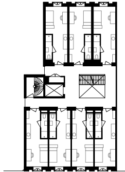
verdieping
