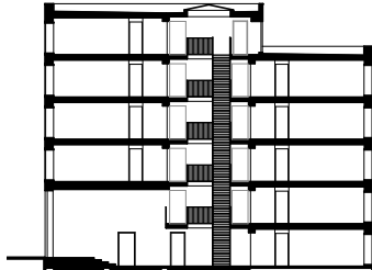
doorsnede
