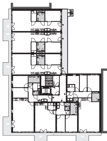
tweede verdieping
