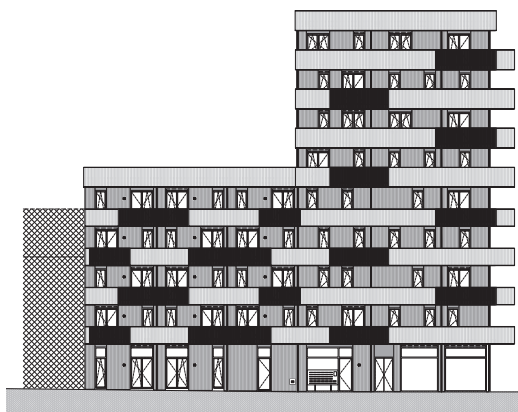
noordwestgevel
