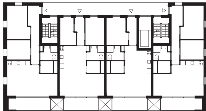
eerste verdieping
