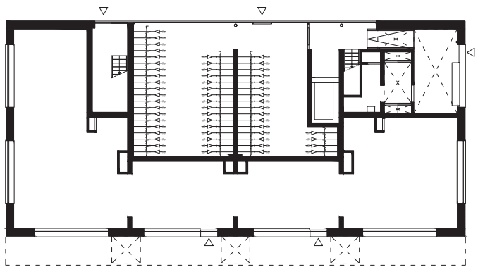
begane grond
