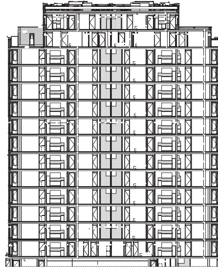
doorsnede toren
