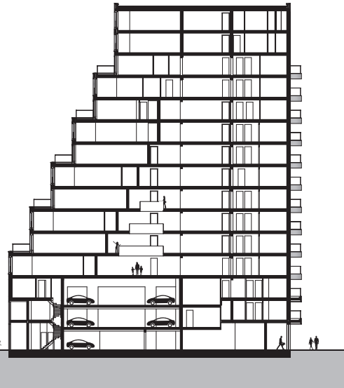
doorsnede
