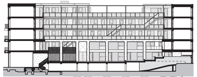
doorsnede
