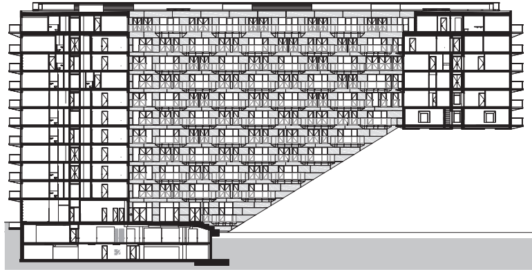
doorsnede
