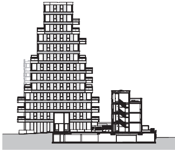
doorsnede
