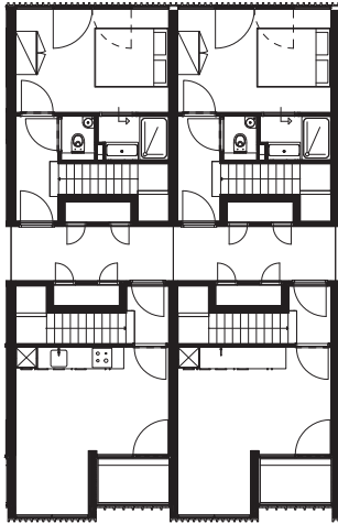
tweede verdieping
