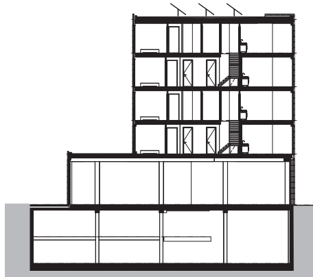
doorsnede
