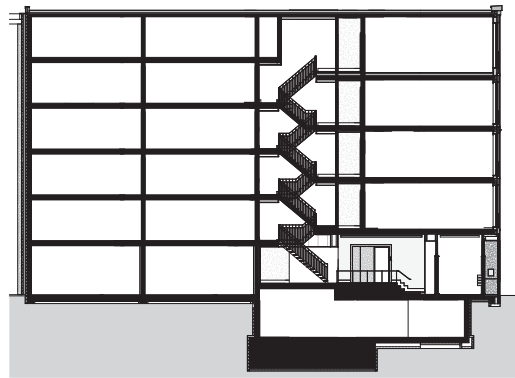
doorsnede
