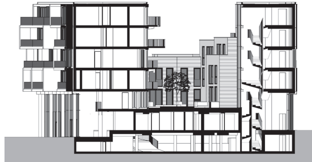
doorsnede
