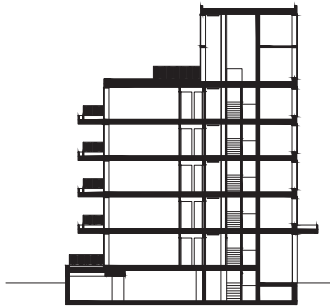
doorsnede
