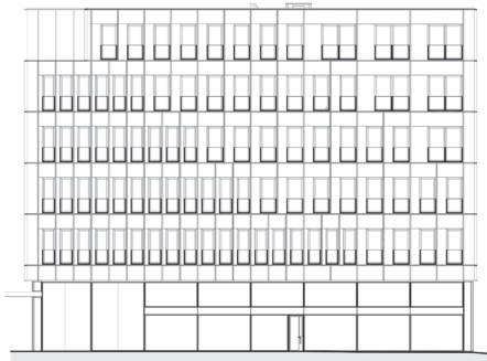
zuidgevel
