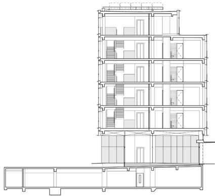
doorsnede
