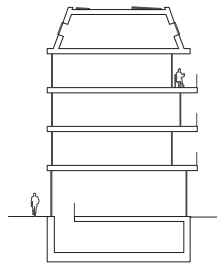
Marnixstraatblok doorsnede
