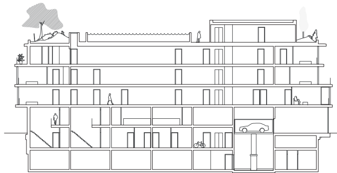
Singelgrachtblok doorsnede
