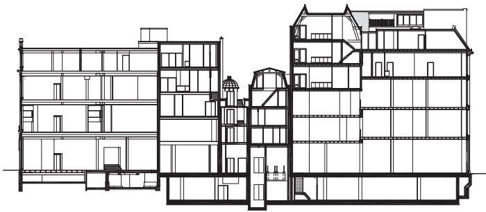
doorsnede
