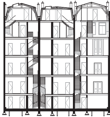
doorsnede
