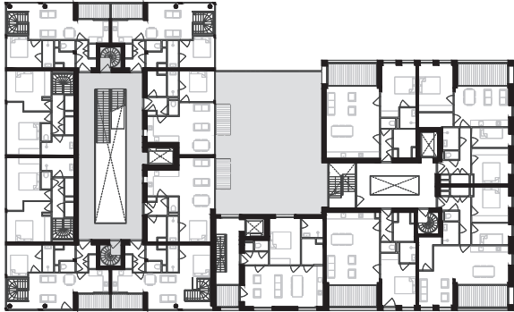
eerste verdieping
