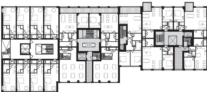
eerste verdieping
